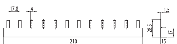
S2L-210-10, S2L-210-16
