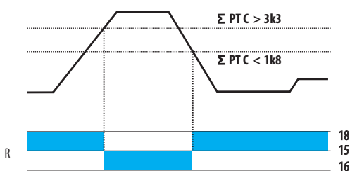
Контроль температуры обмотки двигателя MMR-T1-001-A230
