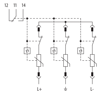
SVC-DC-...-3V-MZS
