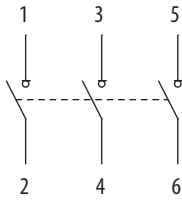
MSN...-3
