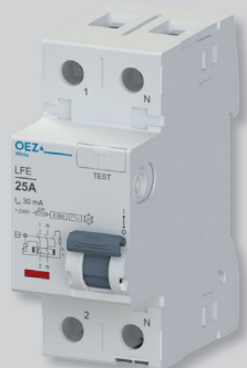
LFE-25-2-030AC
