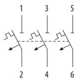
LVN-...-3
