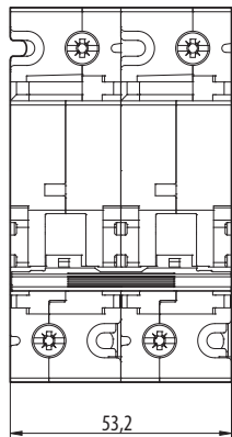
LVN-DC-...-2
