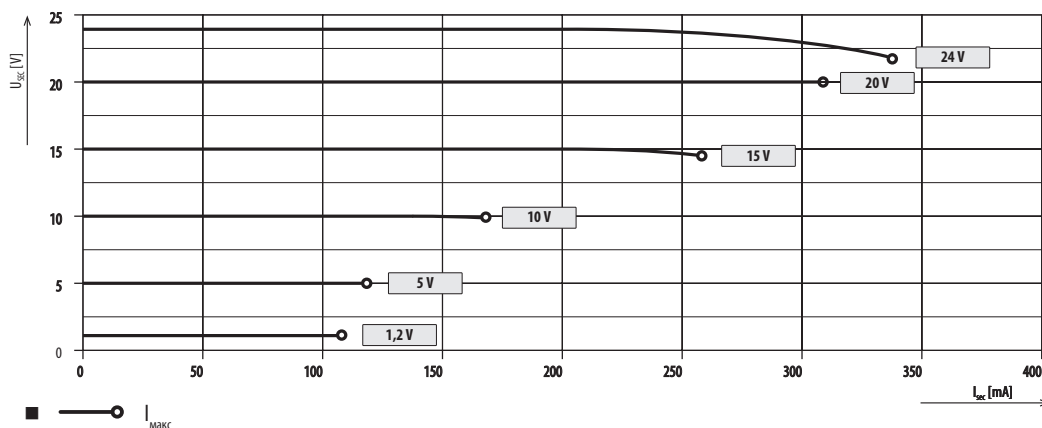
Нагрузочная характеристика UNZR-10T-X024-DC выход
