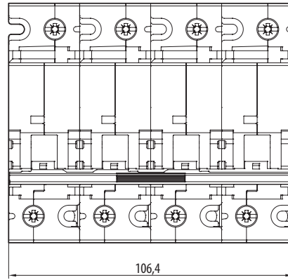
LVN-...-4
